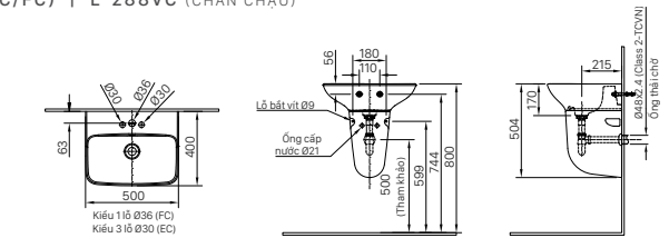
L-289V (EC/FC) | AL-289V (EC/FC) | L-288VC (CHÂN CHẬU)
