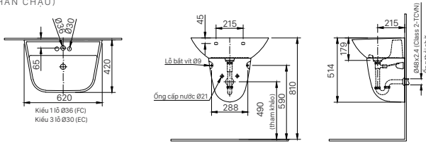
L-289V (EC/FC) | AL-289V (EC/FC) | L-288VC (CHÂN CHẬU)
